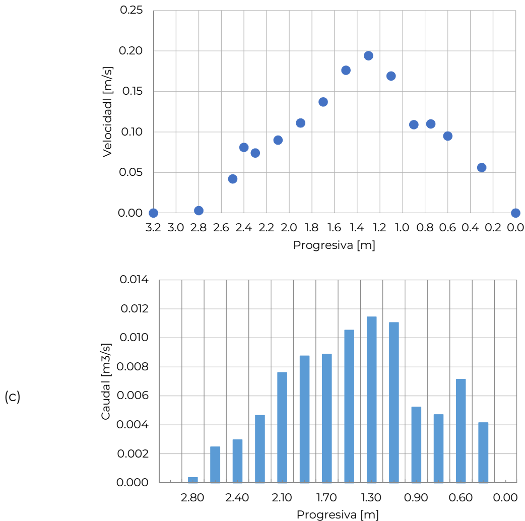
Figura 4.- (a) Sección transversal del arroyo Las Mojarras en el sitio de medición, (b) perfil de velocidades medido y (c) caudal aforado. La progresiva 0,00 se corresponde con la margen derecha.
