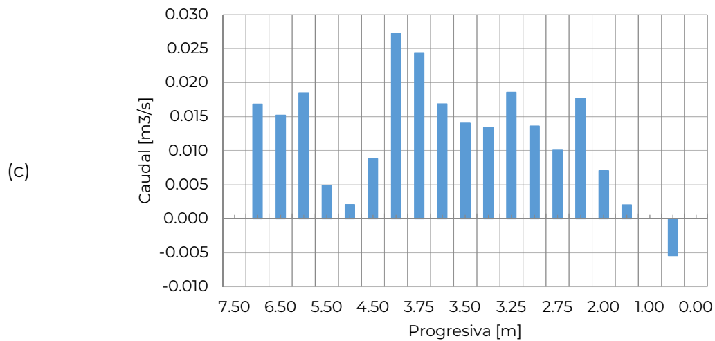
Figura 5.- (a) Sección transversal del arroyo Los Chorrillos en el sitio de medición, (b) perfil de velocidades medido y (c) caudal aforado. La progresiva 0,00 se corresponde con la margen derecha.
