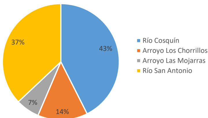
Figura 7. Caudales aportados por ríos tributarios al embalse San Roque, el día 28/05/2024.
