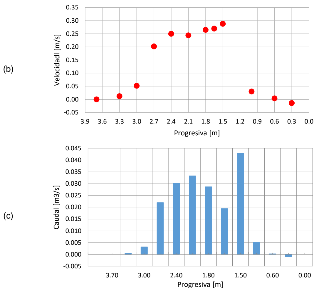
Figura 4. (a) Sección transversal del arroyo Las Mojaras en el sitio de medición, (b) perfil de velocidades medido y (c) caudal aforado con ADC OTT. La progresiva 0.00 se corresponde con la margen derecha.
