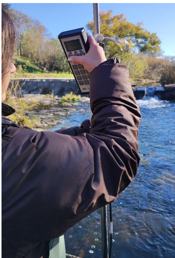
Figura A4. Aforo del arroyo Las Mojarras el día 28/05/2024. Vista aguas arriba
