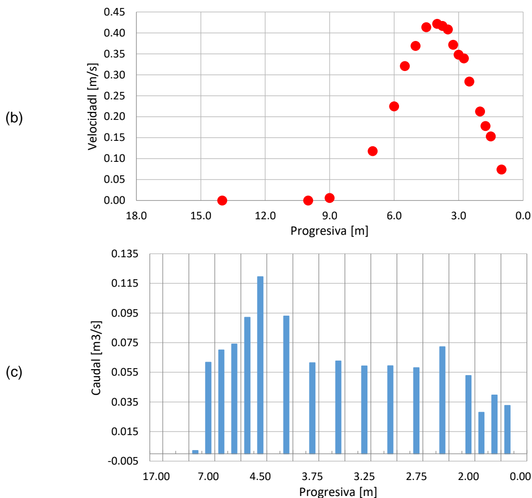
Figura 6. (a) Sección transversal del río San Antonio en el sitio de medición, (b) perfil de velocidades medido y (c) caudal aforado con ADC OTT. La progresiva 0.00 se corresponde con la margen derecha.
