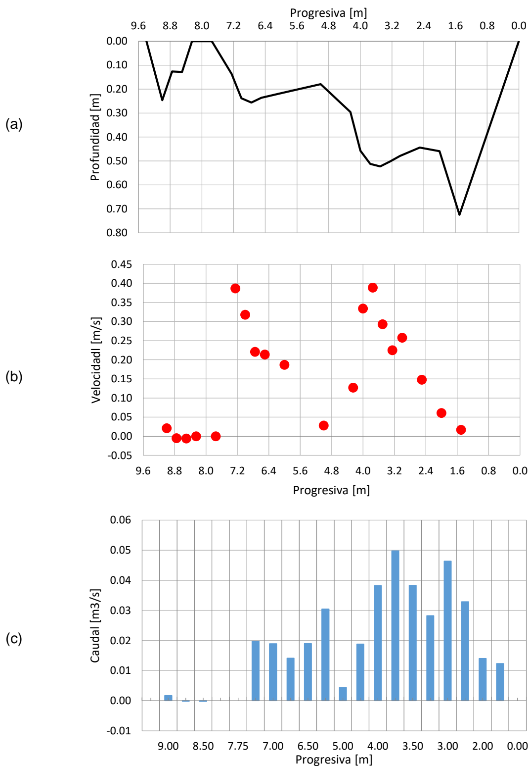
Figura 5. (a) Sección transversal del arroyo Los Chorrillos en el sitio de medición, (b) perfil de velocidades medido y (c) caudal aforado con ADC OTT. La progresiva 0.00 se corresponde con la margen derecha.
