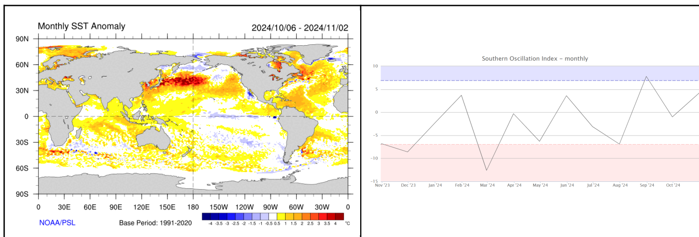
Figura 1: A la izquierda, Anomalía de la temperatura superficial del mar (06-10-2024 al 02-11-2024). Período de referencia 1991-2020 - Fuente: NOAA-NCEP/CPC. A la derecha, Índice SOI mensual . Fuente: Commonwealth of Australia 2018, Bureau of Meteorology (ABN 92 637 533 532)
