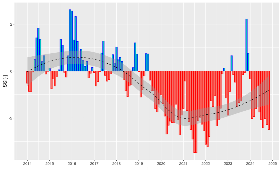
Figura 14: Índice estandarizado de caudal mensual para el río Paraná en Corrientes (período de referencia 1991-2020)
