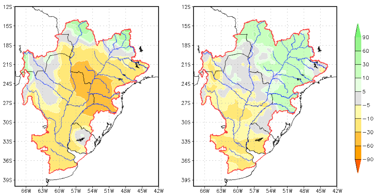
Figura 6: Pronóstico numérico de la anomalía de la precipitación acumulada semanal (mm, somb.) respecto a la climatología del modelo EGFS (2000-2019) para la semana 1 (11/11 al 18/10 12 UTC) y la semana 2 (18/11 al 25/11 12 UTC) .
